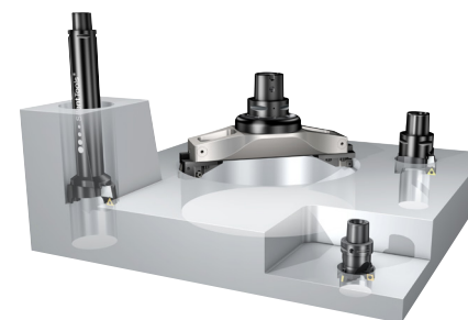
Mandrilamento produtivo Mandrilamento escalonado* Mandrilamento de aresta única*
