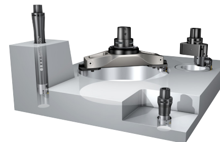
通常ボーリング バックボーリング* 外径ボーリング
