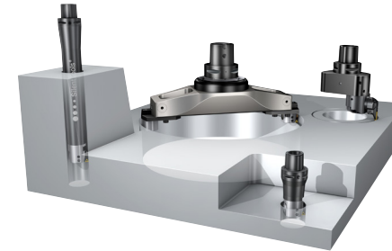
Herkömmliches Aufbohren
