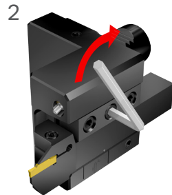
Soltar el mango de herramienta
