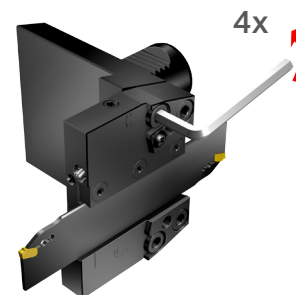
Einstellen der Mittenhöhe
