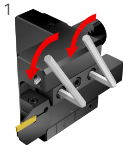
Soltar el mango de herramienta
