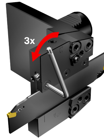
Einsatz zum Abstechen lösen
